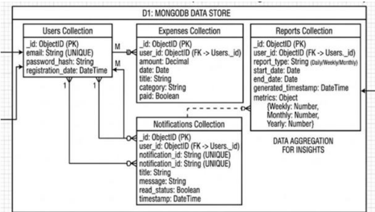
Figure 4.6: ER Diagram
